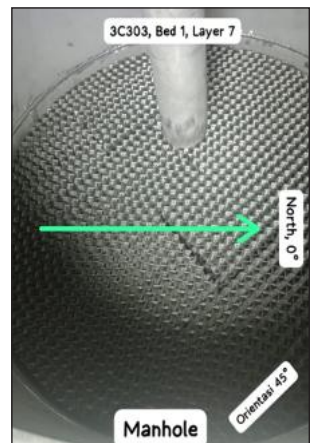
Manhole
