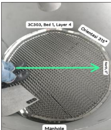
Manhole
