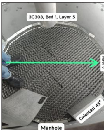
Manhole
